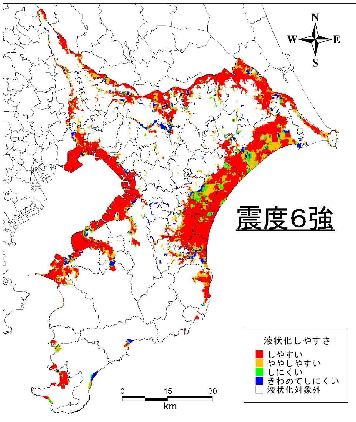
図 液状化しやすさマップ (巨大地震・震度6強・地表加速度960gal)
